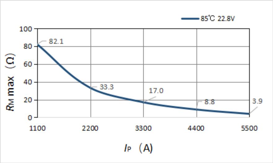
图 2 测量电阻
