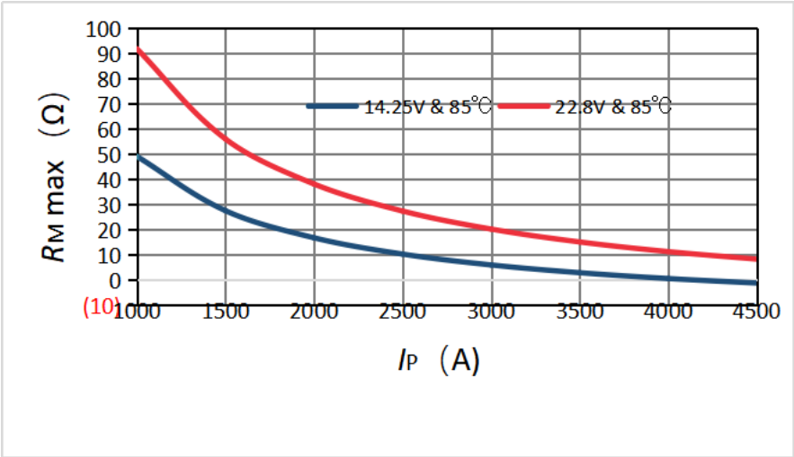
图 1 测量电阻
