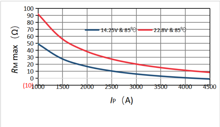
图 1 测量电阻
