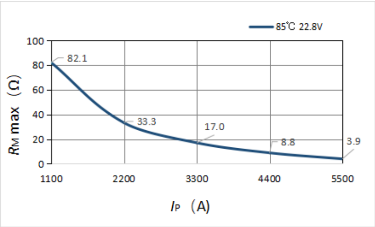
图 1 测量电阻
